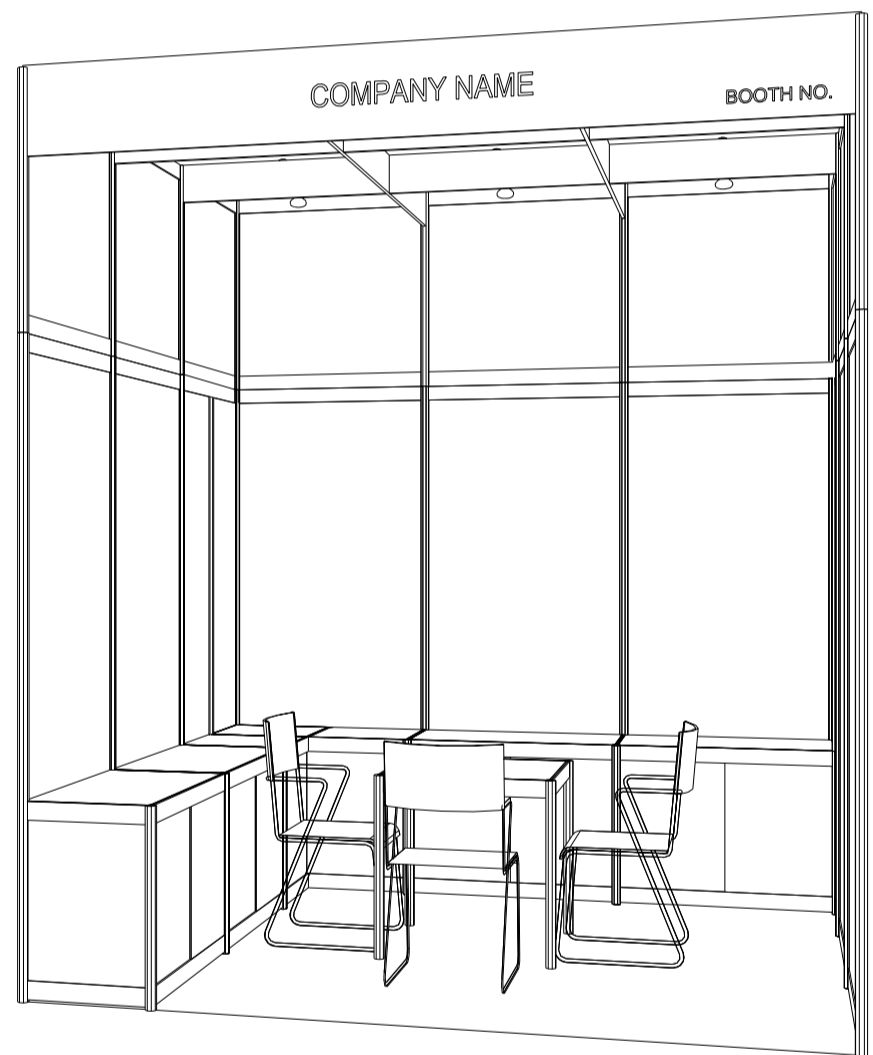
PERSPECTIVE 3M(W) X 3M(D) X 3.5M(H)
